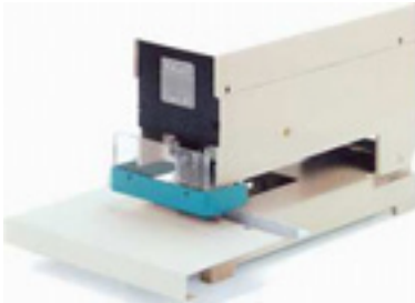
Tak - 18 Grapado en plano para confección de talonarios. Accionamiento a pedal. Capacidad 160 hojas/80 gramos.
